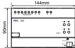
KNX 4CH 1.5A MOSFET Dimming Actuator
