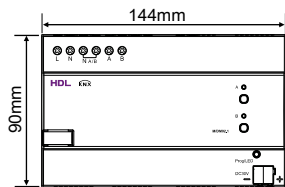
KNX 2CH 3A MOSFET Dimming Actuator
