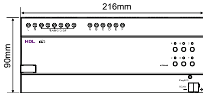
KNX 6CH 1.5A MOSFET Dimming Actuator
