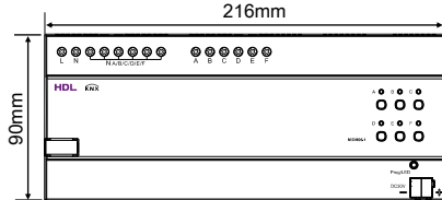
KNX 6CH 1.5A MOSFET Dimming Actuator
